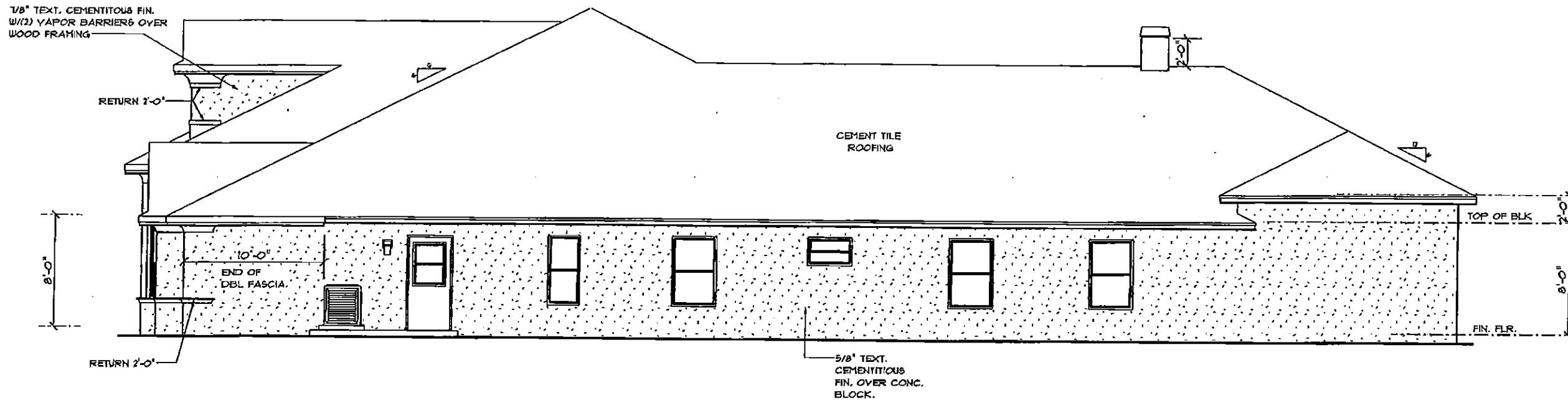
RIGHT ELEVATION
